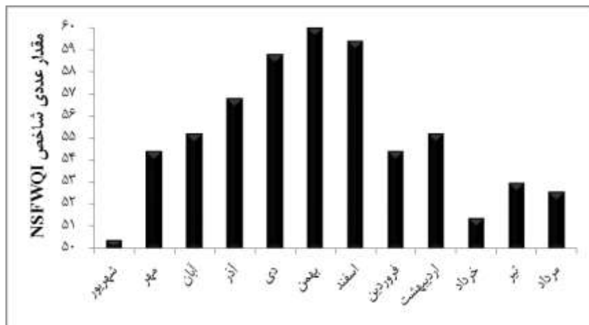
شکل ۴: میانگین شاخص NSF-WQI در ماه‌های مورد مطالعه.
