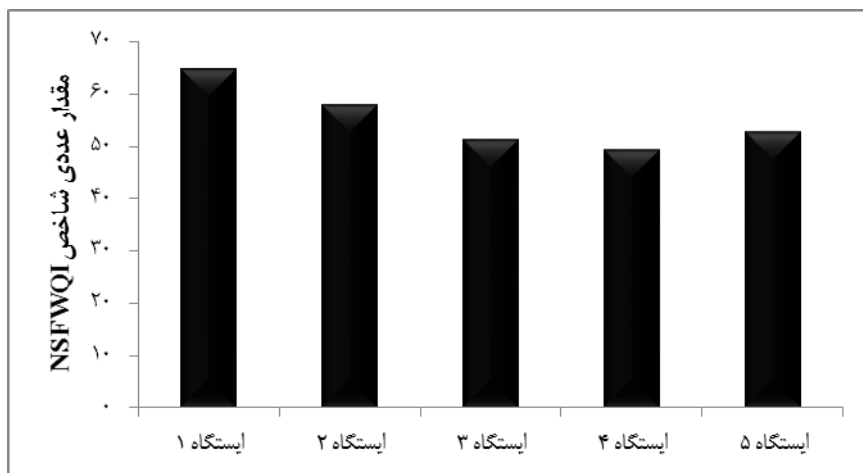
شکل ۲: میانگین شاخص NSFQI در ایستگاه‌های مورد مطالعه.
