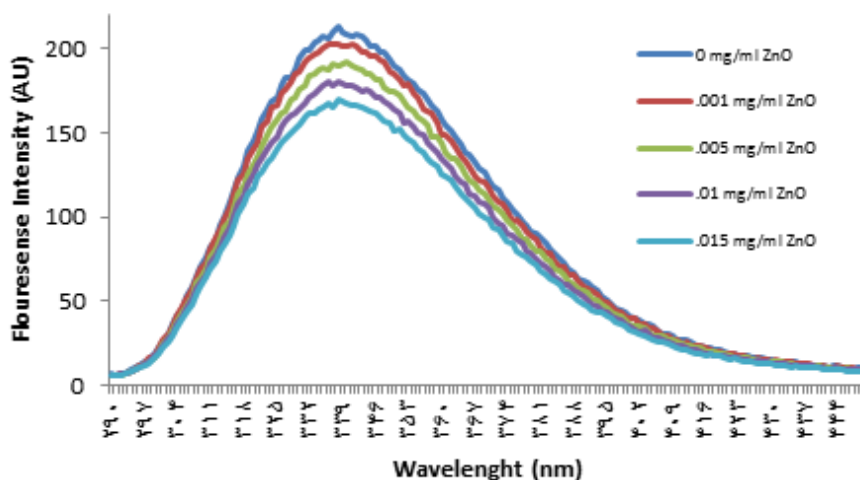
شکل 6. a. تغییرات نشر فلورسانس آنزیم لیزوزیم در حضور غلظت‌های مختلف نانوذره ZnO در pH 7 و دمای ۲۵°C
