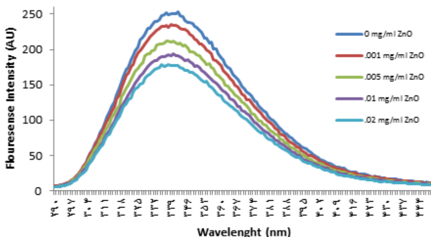
شکل 6. b. تغییرات نشر فلورسانس آنزیم لیزوزیم در حضور غلظت‌های مختلف نانوذره ZnO در pH 7 و دمای ۳۵°C
