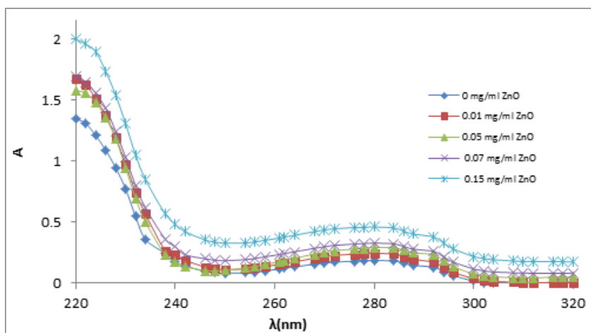
شکل ۳. تغییرات جذب ۲۸۰ نانومتر در مقابل غلظت‌های مختلف نانو ذره ZnO
