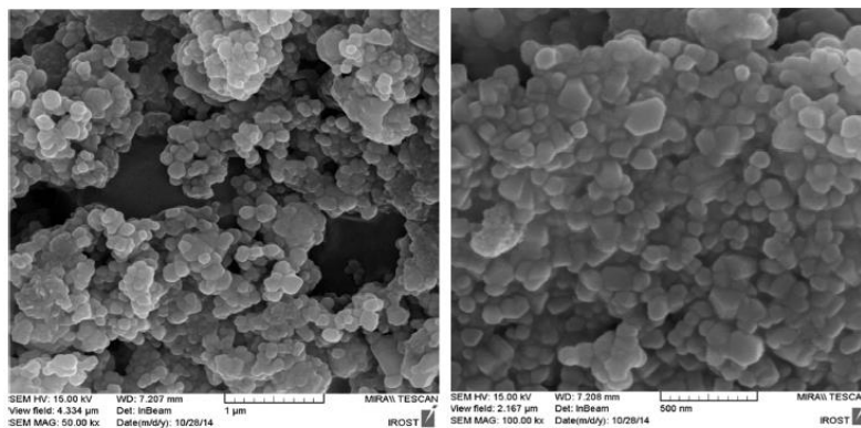
شکل ۱. تصویر میکروسکوپ الکترونی نانوذره ZnO
