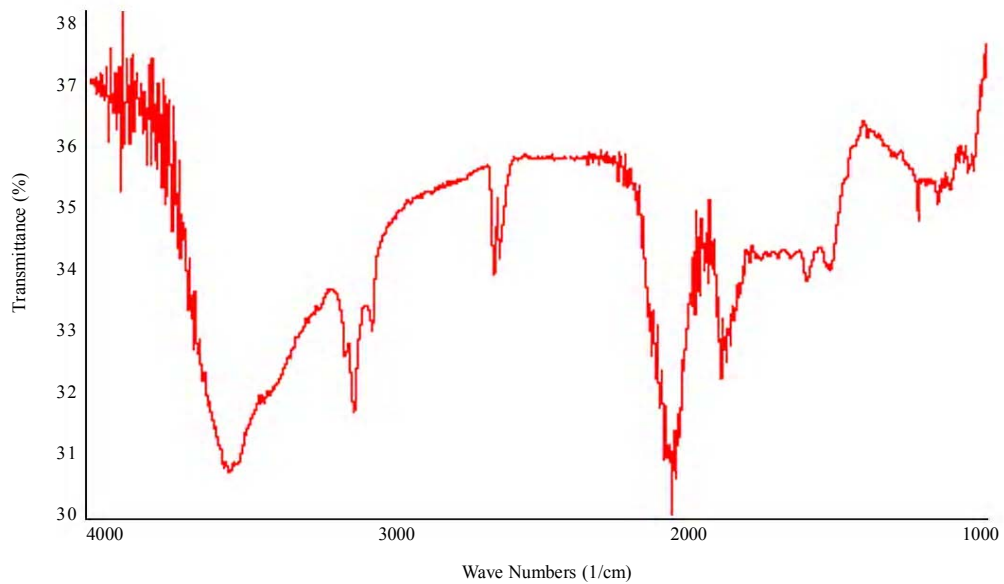
Fig. 3: FTIR spectra of BS of N. otitidiscaviarum
