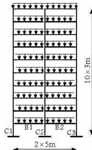
شکل ۴- مشخصات هندسی قاب ده طبقه
