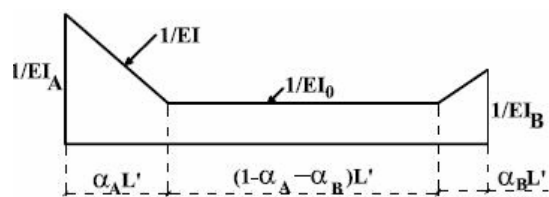
شکل ۳- نمودار نرمی خمشی عضو بتنی در حالت غیرخطی
